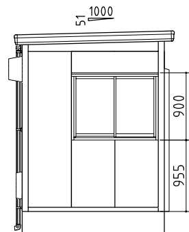
左側面図
