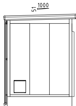
左側面図
