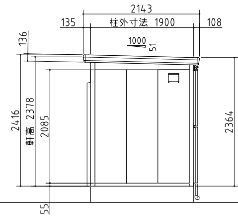
右側面図
