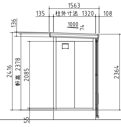
右側面図
