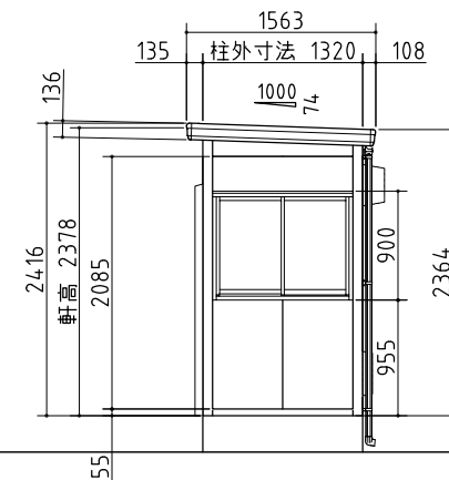
右側面図
