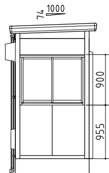
左側面図
