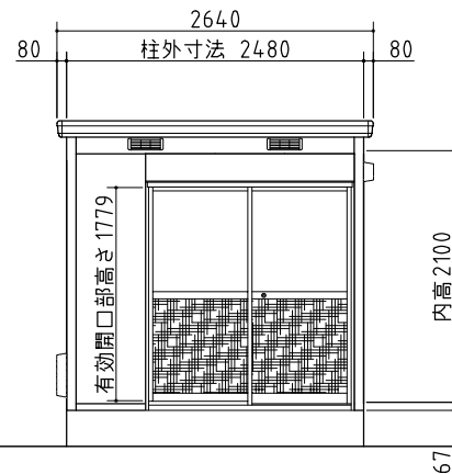
正面図
