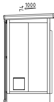
左側面図
