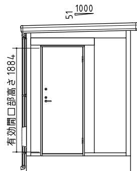
左側面図
