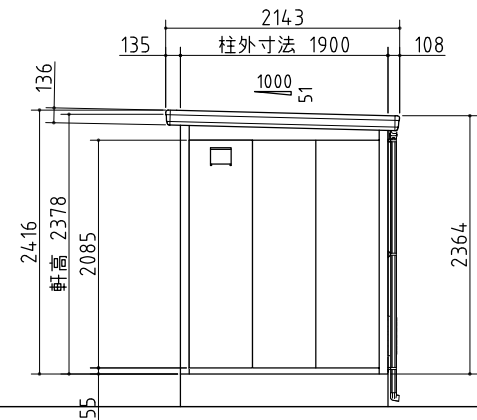
右側面図
