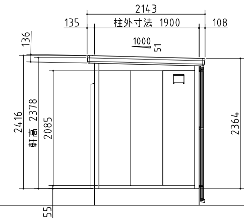
右側面図
