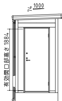
左側面図
