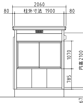
正面図
