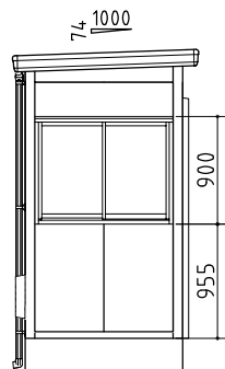
左側面図
