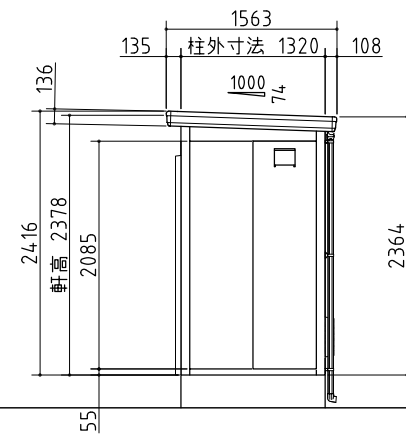
右側面図
