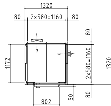
平面図
