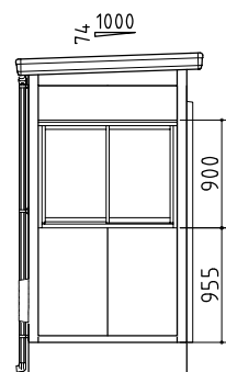
左側面図
