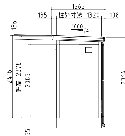
右側面図
