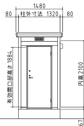
正面図
