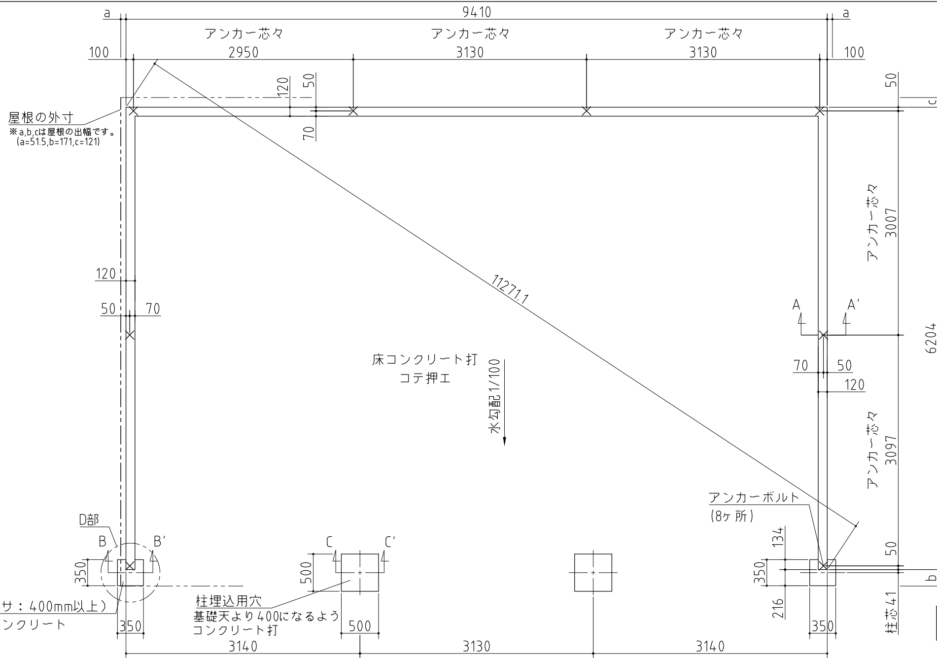
基礎詳細図 S=1/20
