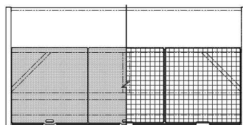
平面断面図
