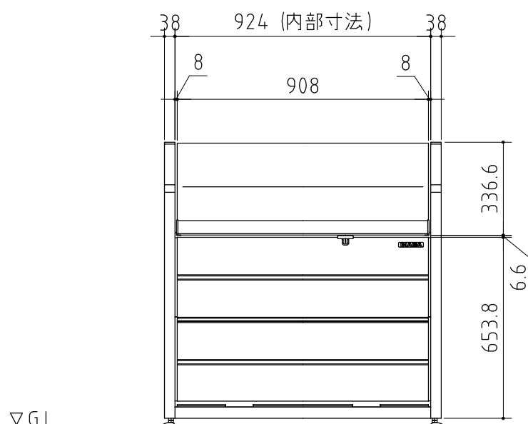
正面図
