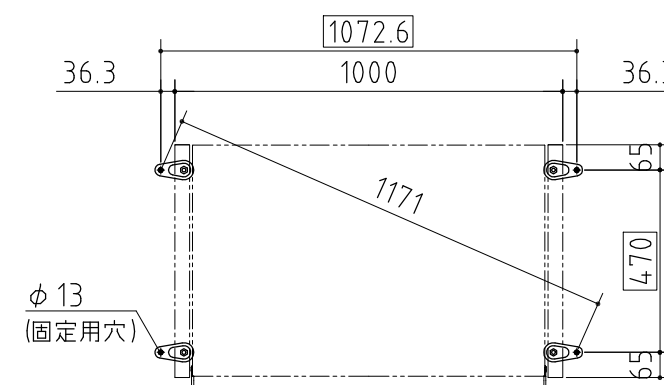
【外側でアンカー固定する場合】
