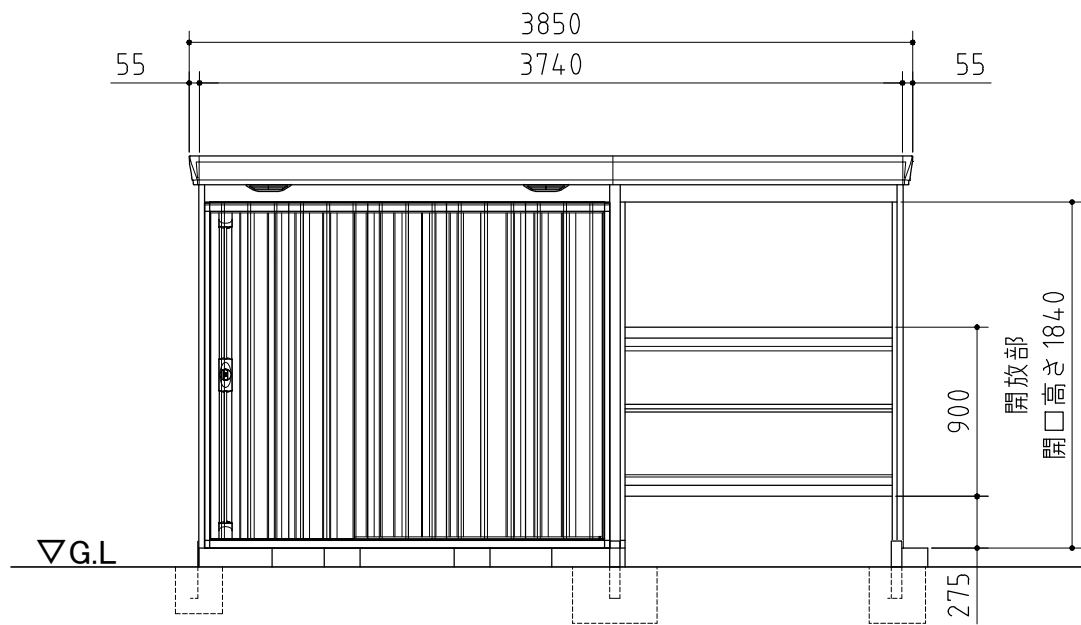
正面図
