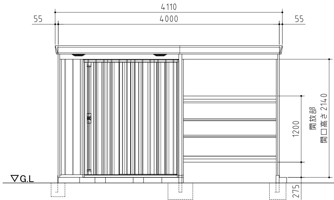
正面図
