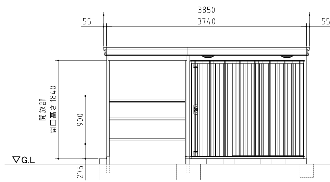
正面図
