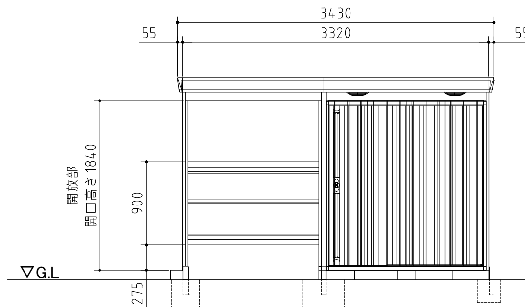
正面図
