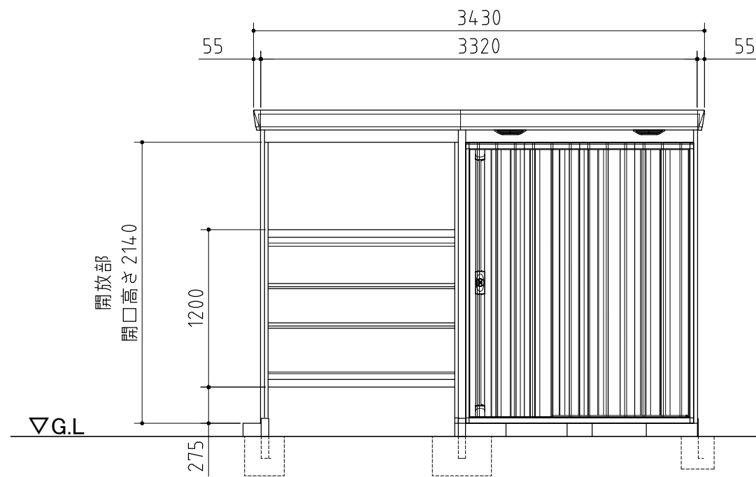
正面図
