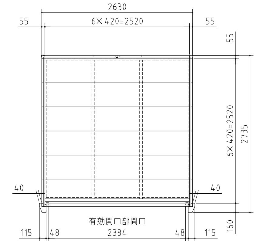
平面図
