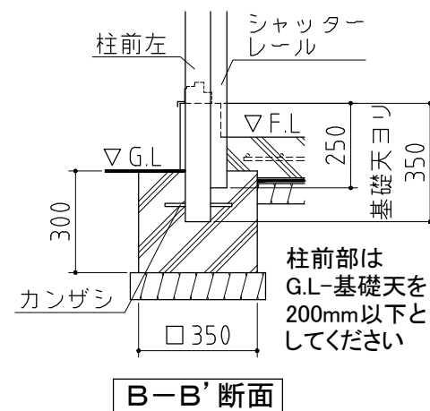
基礎詳細図 S=1/20
