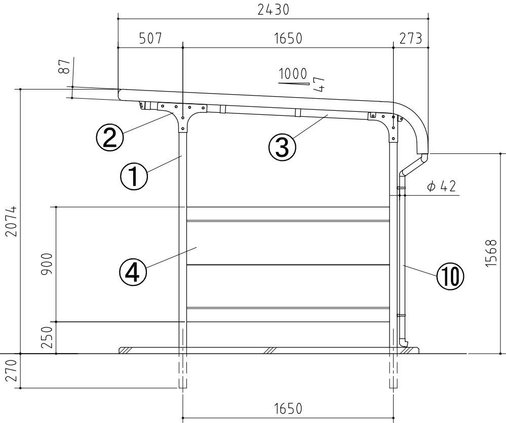
側面図
