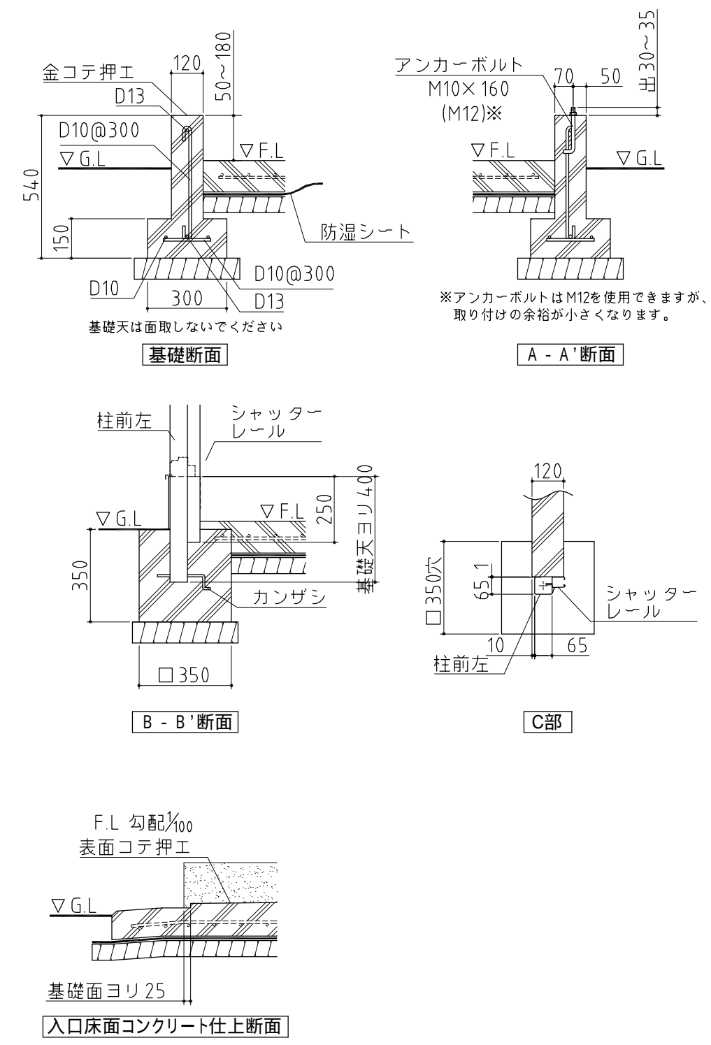
基礎詳細図 S=1/20
