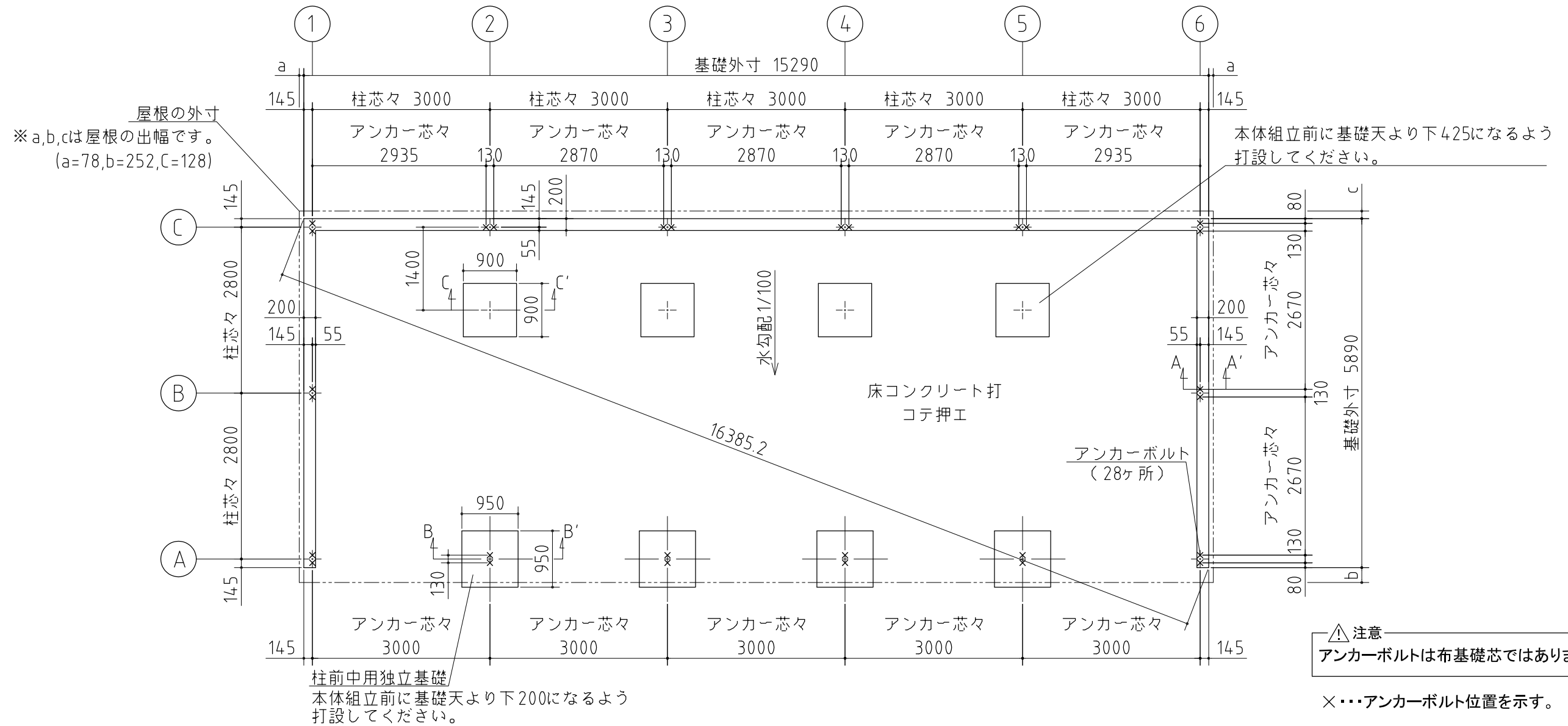
基礎詳細図 S=1/20
