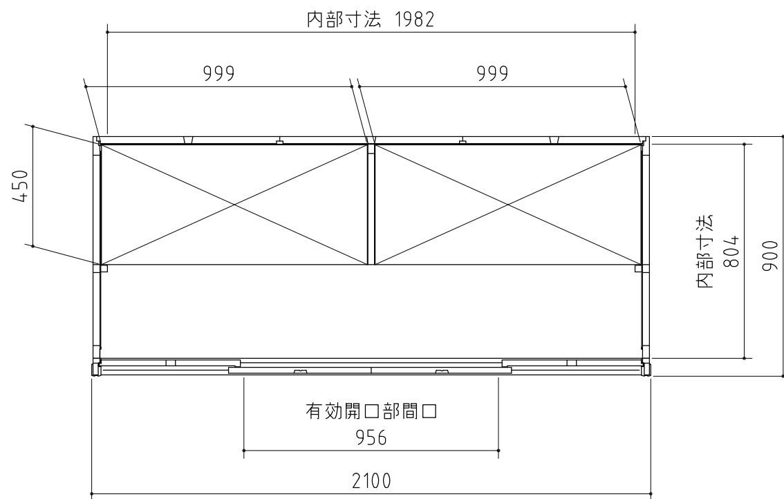
平面図
