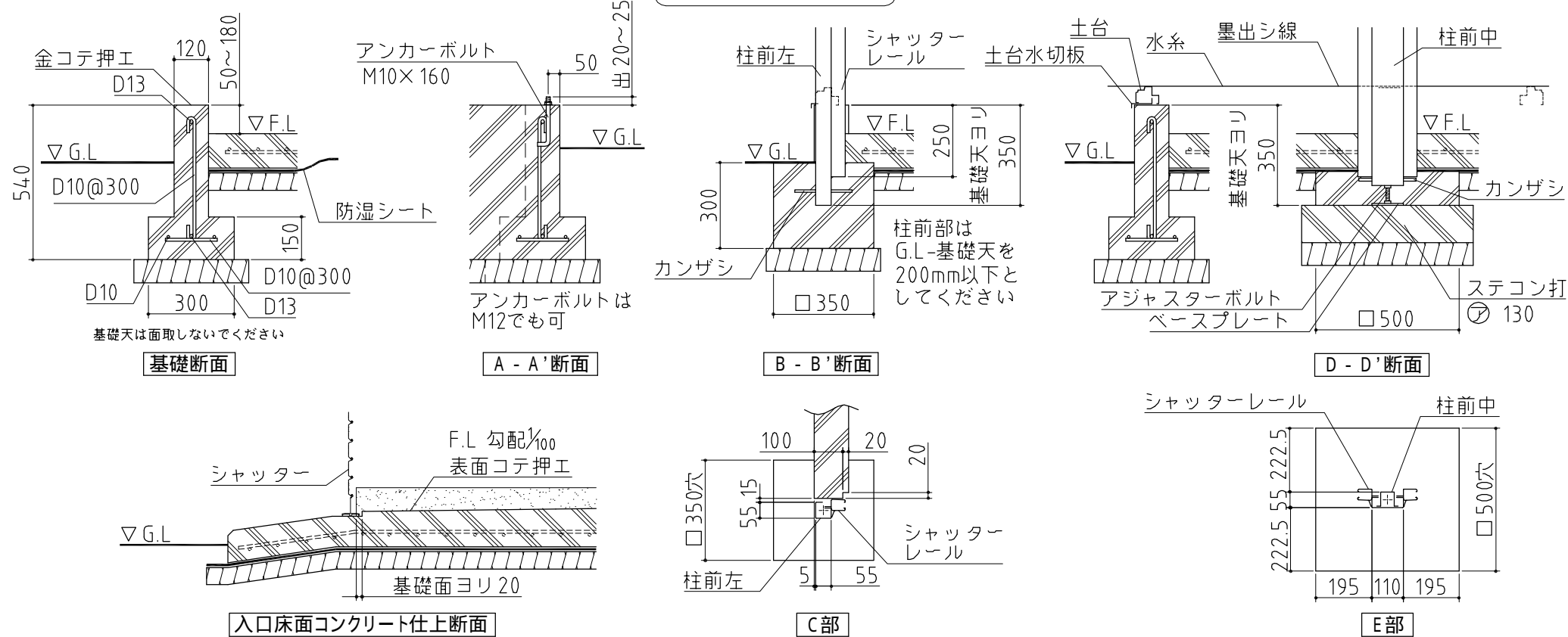
基礎詳細図 S=1/20
