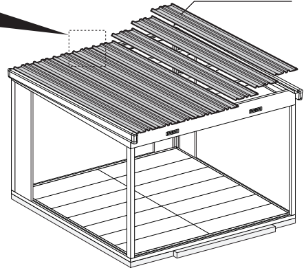
(24)屋根パネル
