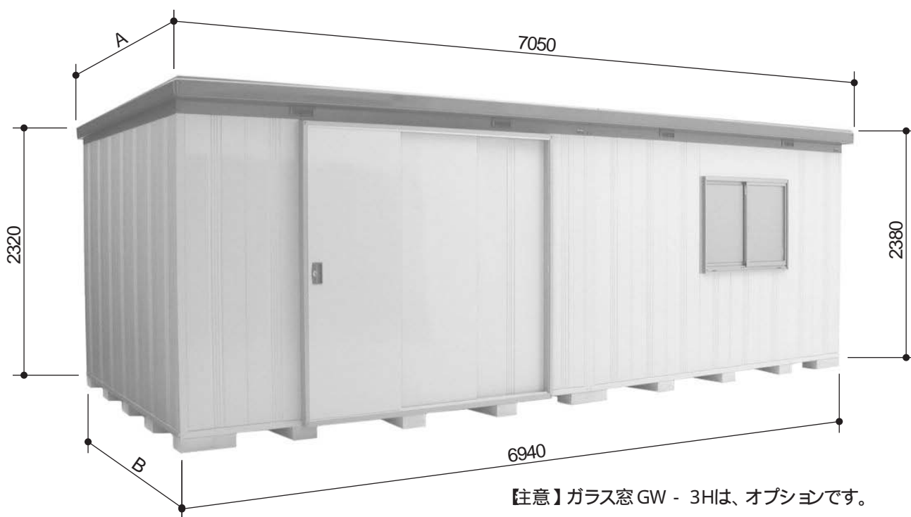
MBW -180H・220H・245H型 寸法図 (写真は、MBW -220H型です。)
