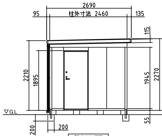
側面図
