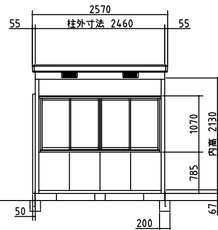
正面図
