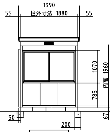
正面図
