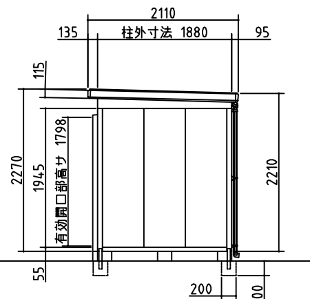
側面図
