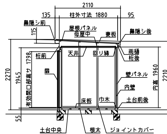
断面図
