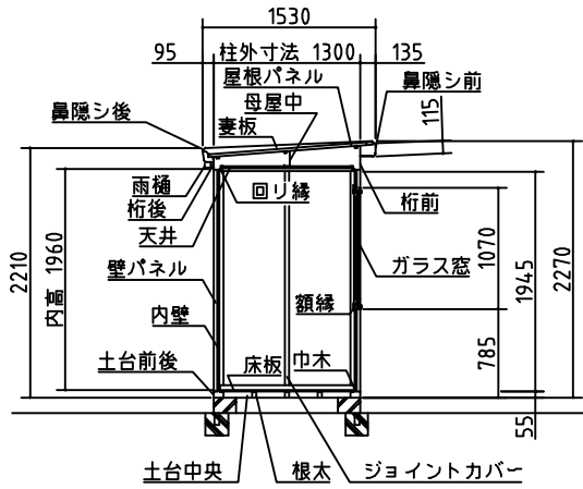
断面図
