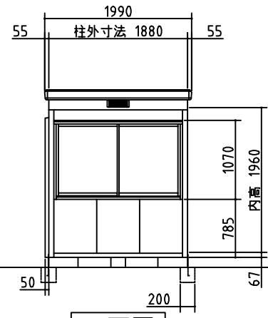
正面図
