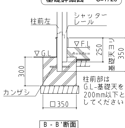
基礎詳細図 S=1/20
