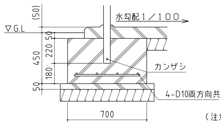
A-A' 断面 1/20
