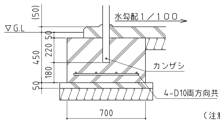
A-A' 断面 1/20
