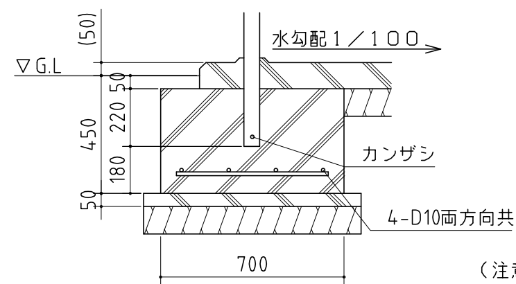
A-A' 断面 1/20
