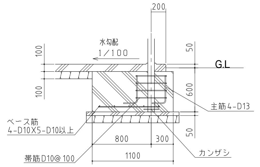
A-A' 断面
