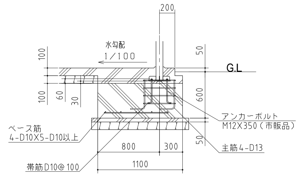
A-A' 断面
