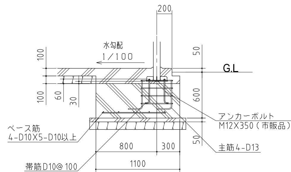
A-A' 断面
