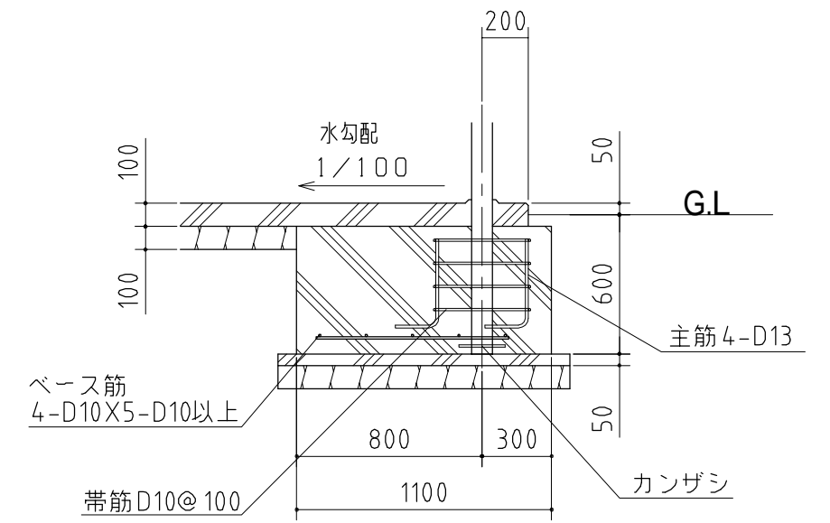
A-A' 断面
