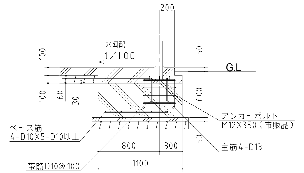
A-A' 断面
